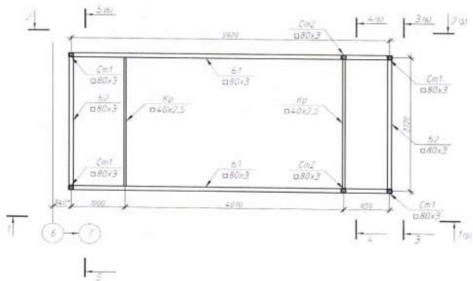
Схема стоек и балок на отм. +2,420
